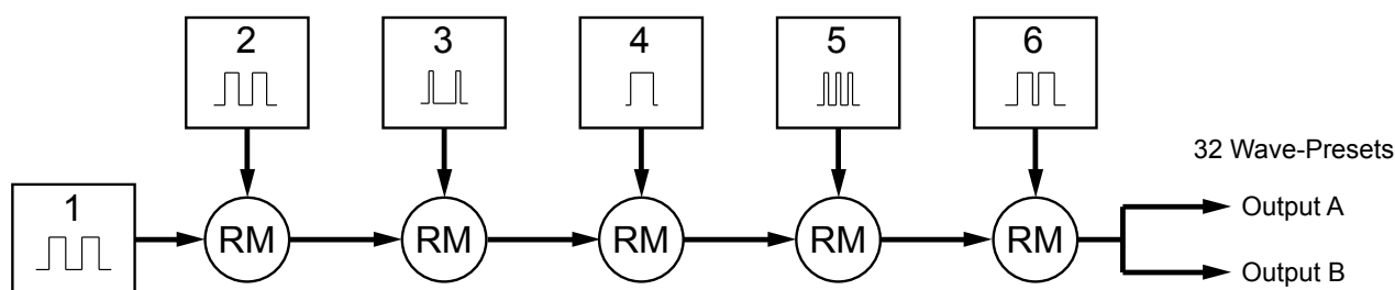
Wellenform- Erzeugung
